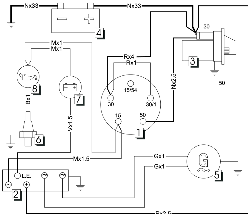
Color x Section (mm 2 ) - Colore x Sezione (mm 2 ) - Couleur x Section (mm 2 ) Farbe x Querschnitt (mm 2 ) - Color x Sección (mm 2 )
